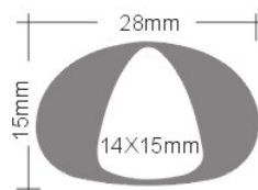
三角形小 Triangle (S)
