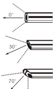
A0010 0° 内窥镜 Endoscope Φ4×302mm
