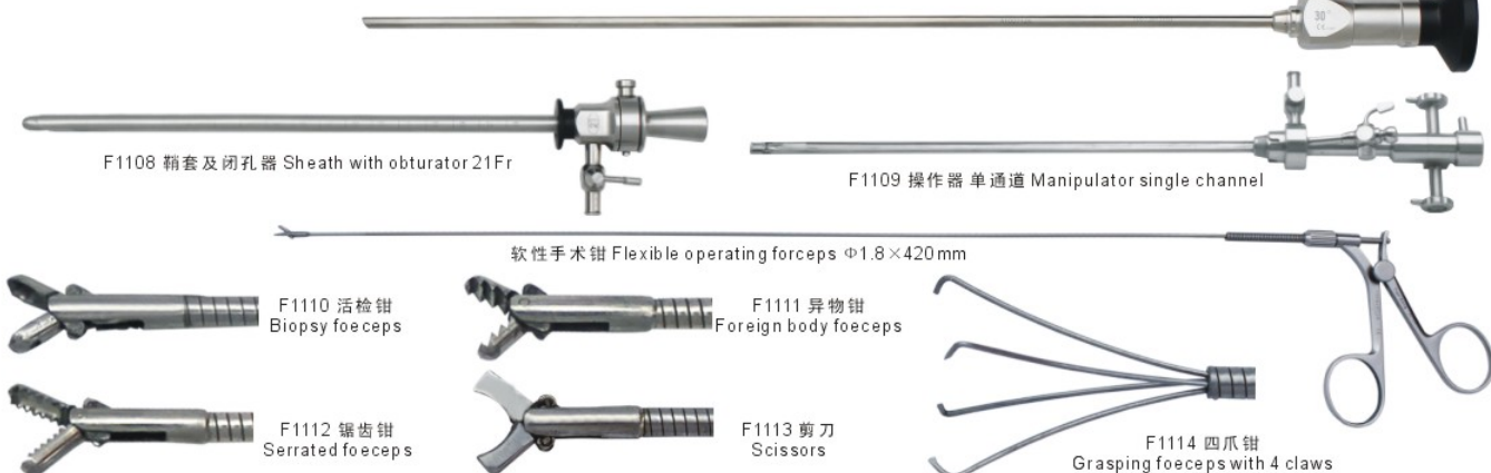
A0012 30° 内窥镜 Endoscope Φ4×302mm
